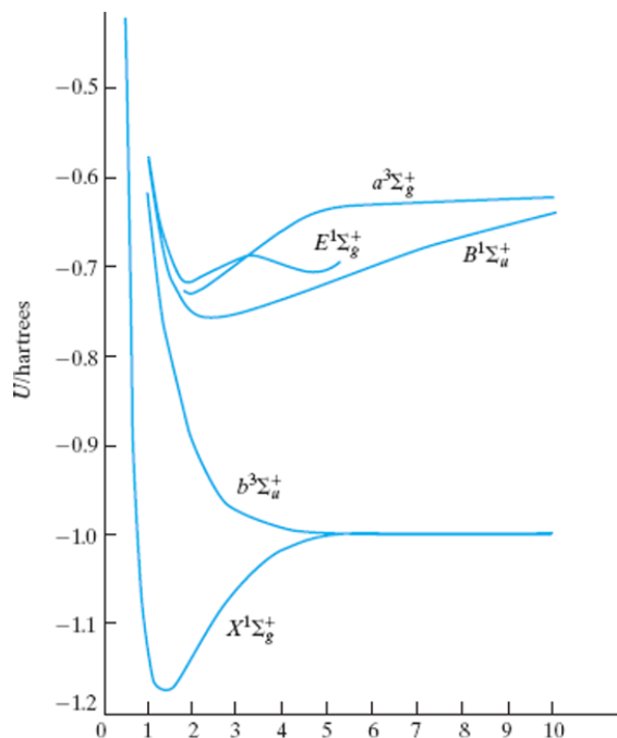
图 13.19: H_2 部分电子态的 U(R) 曲线。【See W. Kolos and L. Wolniewicz, J. Chem. Phys. , 43 , 2429 (1965); 45, 509 (1966); J. Gerhauser and H. S. Taylor, J. Chem. Phys. , 42 , 3621 (1965); W. Kolos, J. Mol. Spectry , 143 , 237 (1990).】
